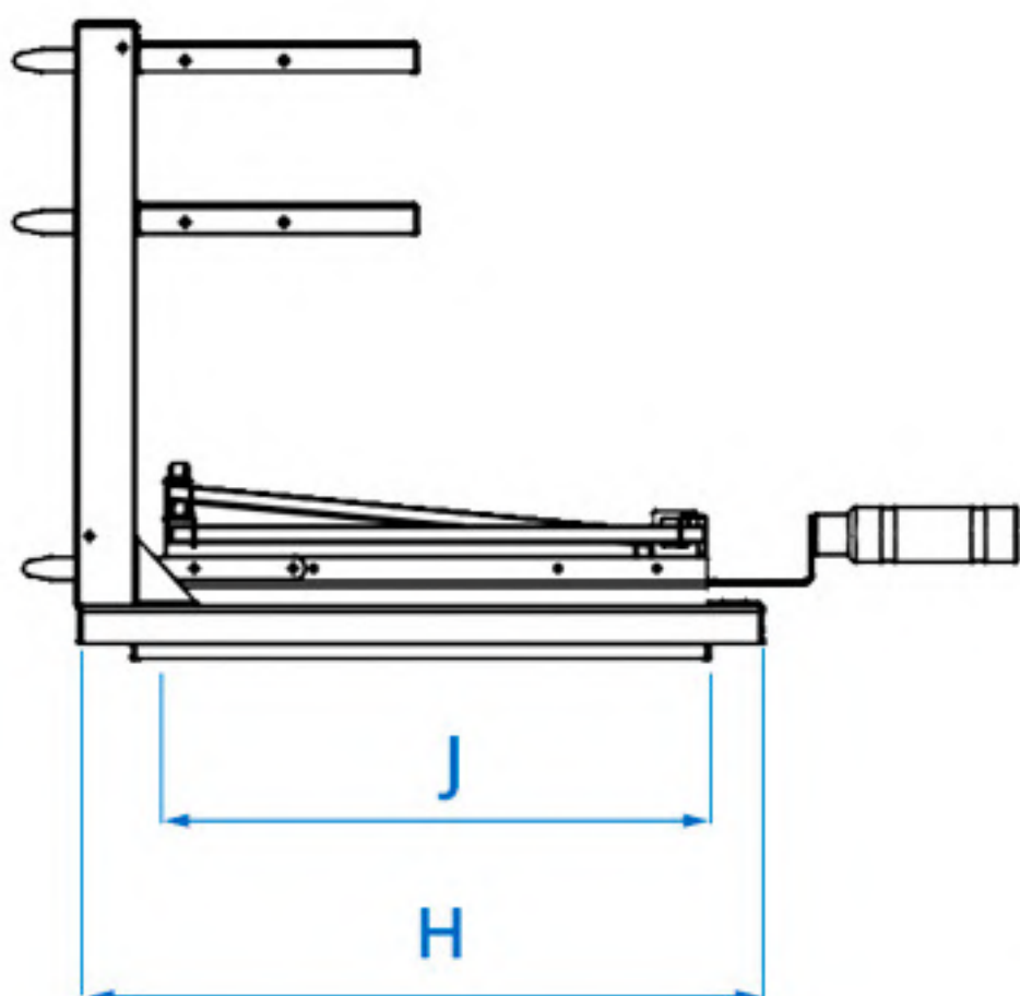
VISTA LATERAL
