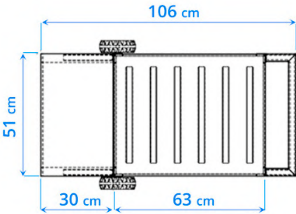
PLANTA (COIFA)
