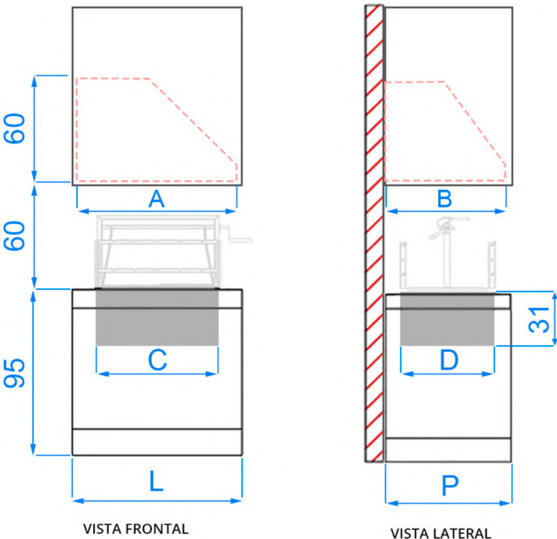
VISTA LATERAL
