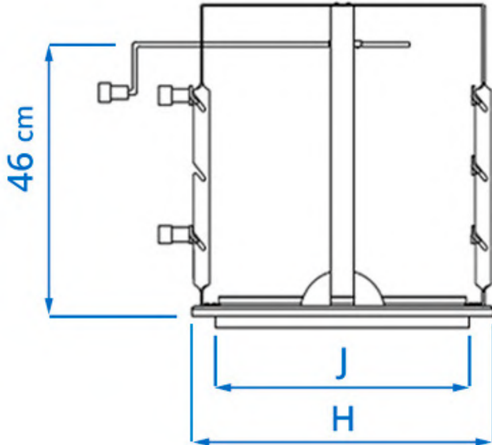
VISTA LATERAL
