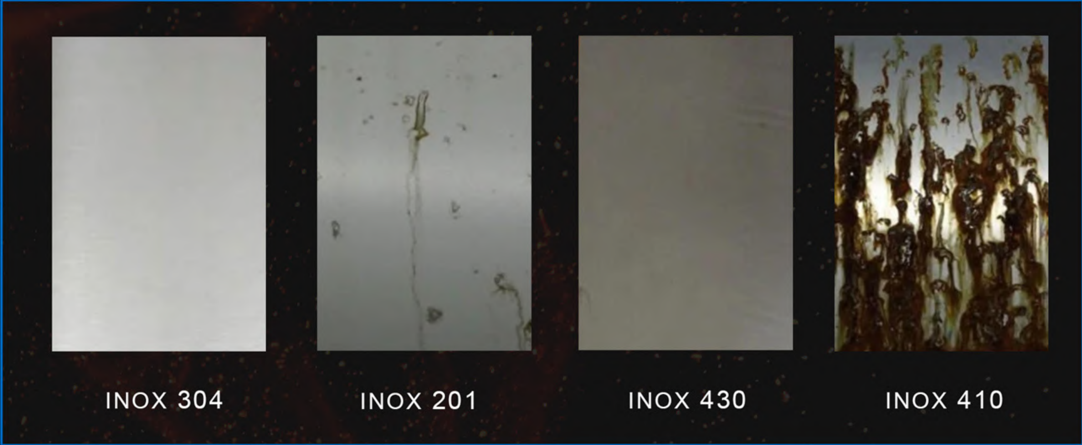
Ensaados após 30 dias de exposição em névoa salina (FONTE: APERAM)
