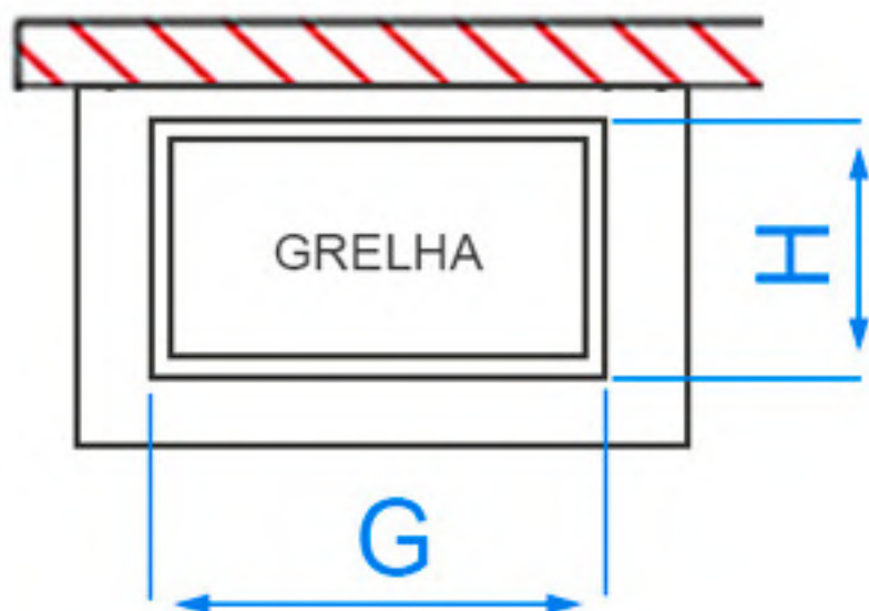
PLANTA (BRASEIRO)
