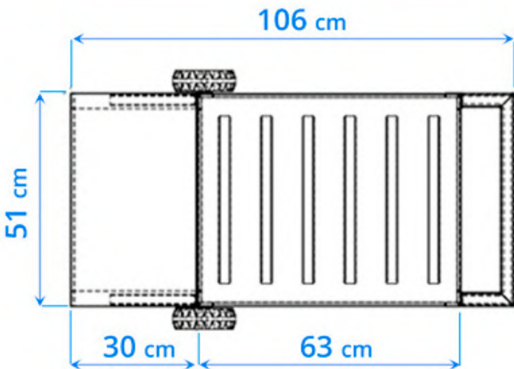
PLANTA (COIFA)
