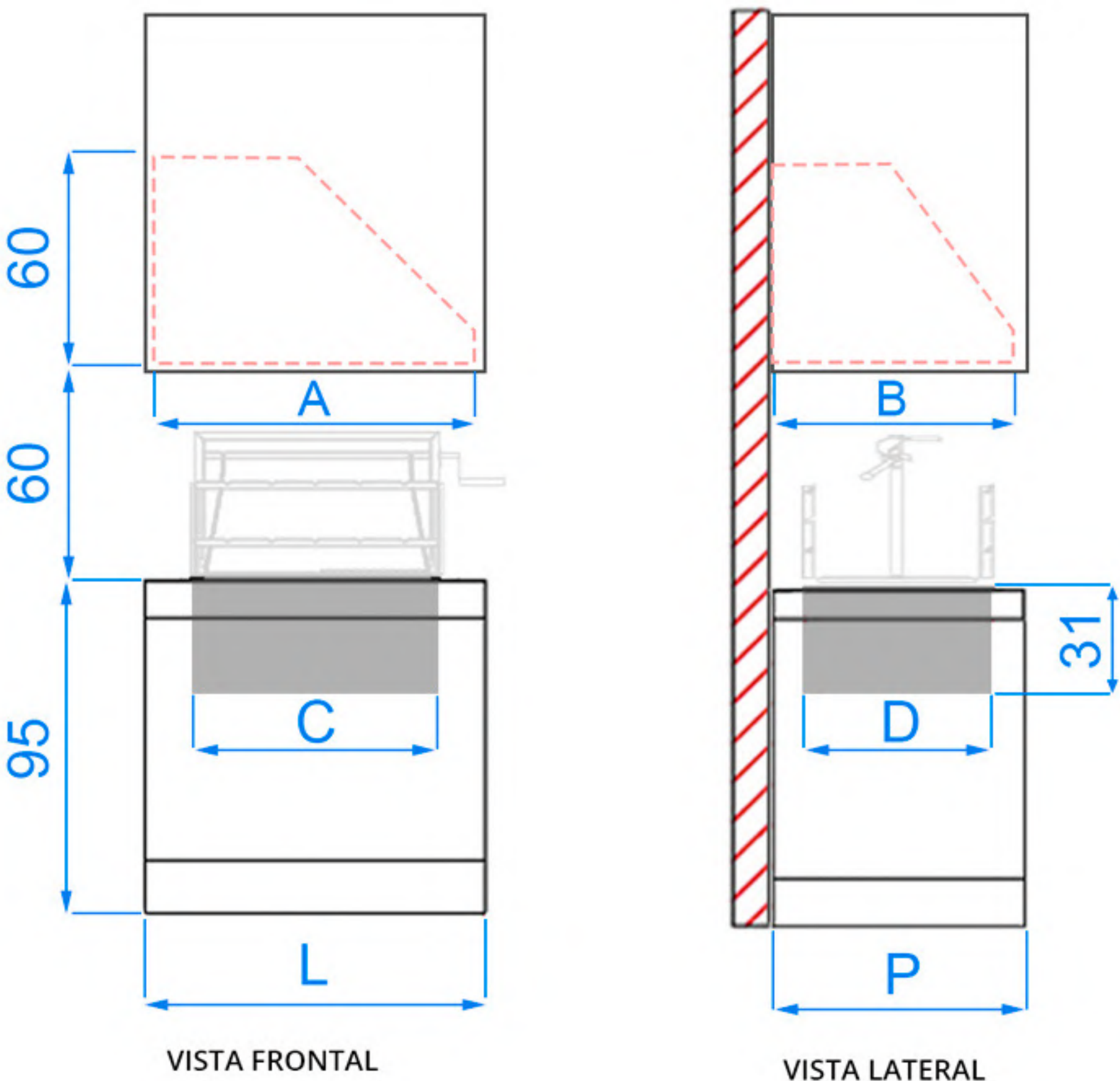
VISTA LATERAL
