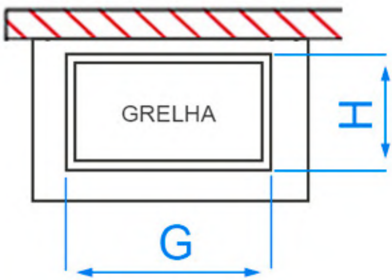
PLANTA (BRASEIRO)
