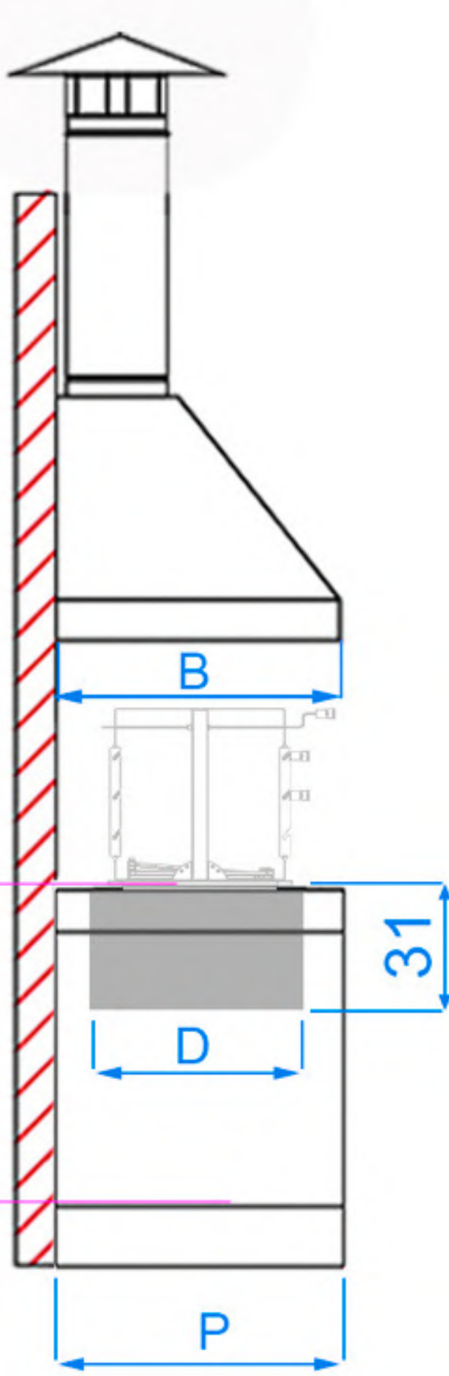
VISTA LATERAL
