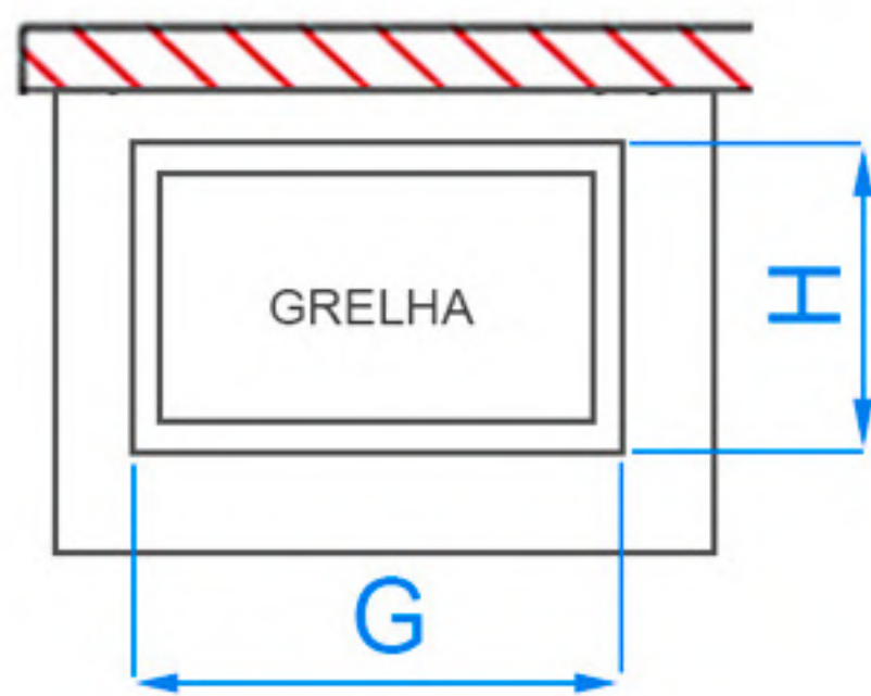
PLANTA (BRASEIRO)
