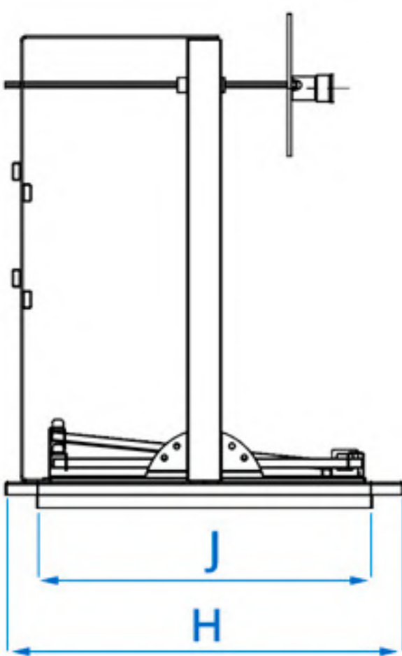
VISTA LATERAL
