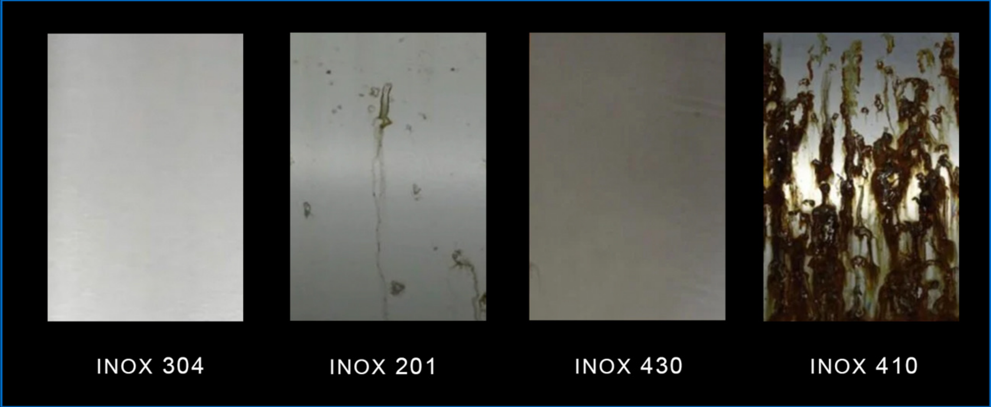
Ensaiaados após 30 dias de exposição em névoa salina (FONTE: APERAM)
